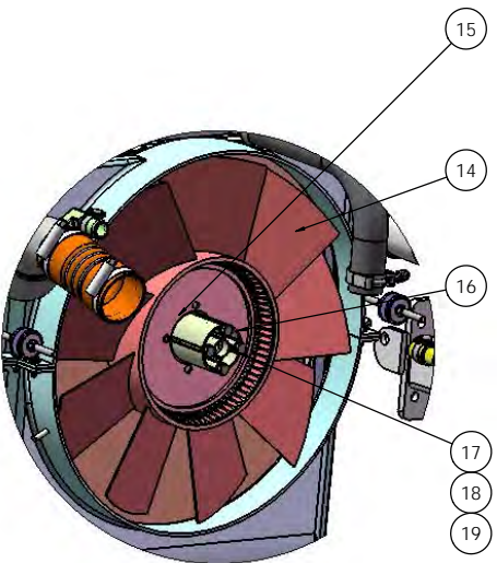
FAN DETAIL
